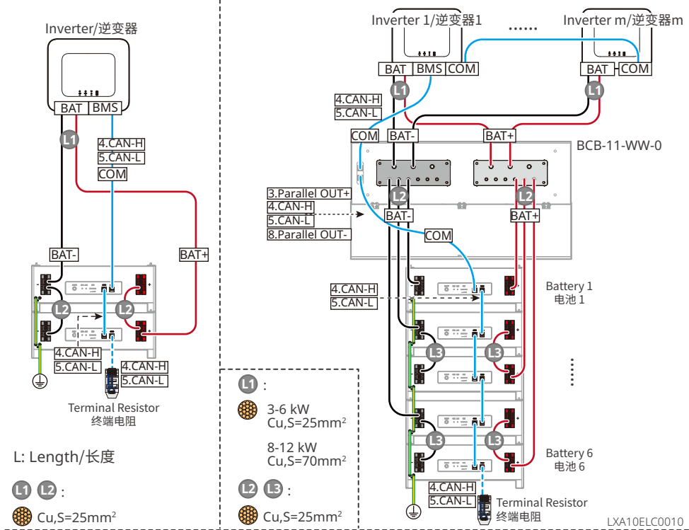
Direct Connection Mode/直连模式
